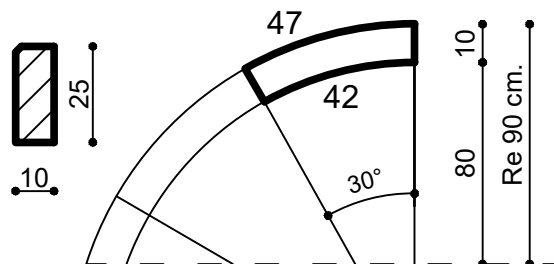
SEZ 10x25 cm Re = 0,9 mt
