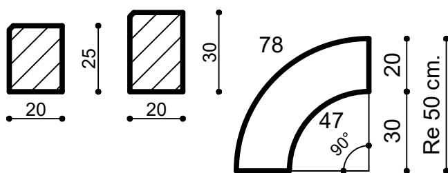
SEZ 20x25 e 20x30 cm Re = 0,5 mt
